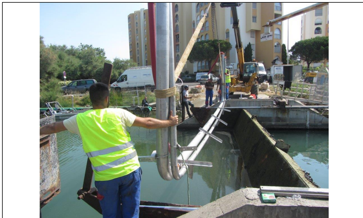
Mise en place de la buse de protection pour les flexibles hydrauliques de la rive gauche
